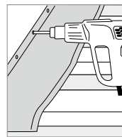
4. Befestigung entlang der Oberkante ohne Dehnung des DEKTITE®.
